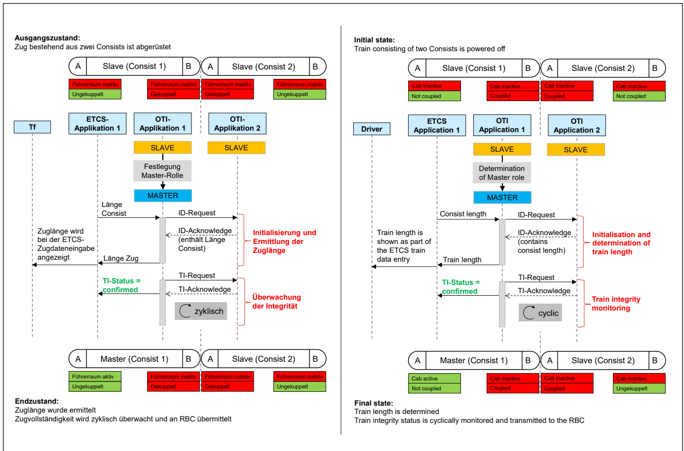
Bild 4: Betriebsszenario "Initialisierung und Ermittlung der Zuglänge" bei einem Zug, der aus zwei gekoppelten Consists besteht
